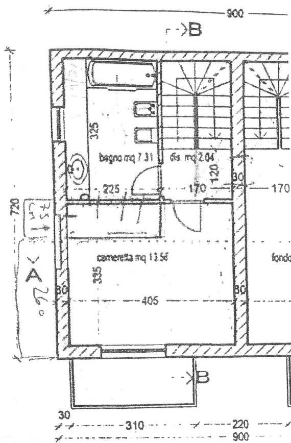
Pianta piano superiore
